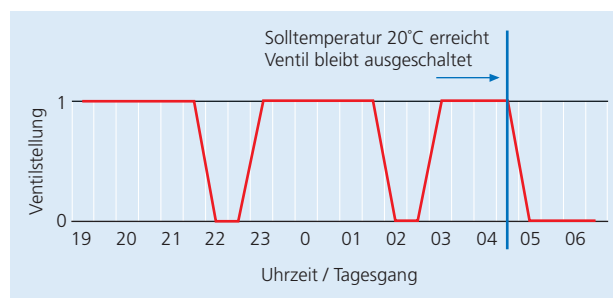
Beton-Entladezyklus
