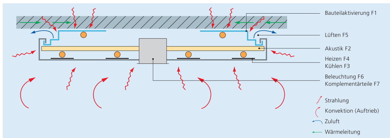
Prinzipanschnitt
