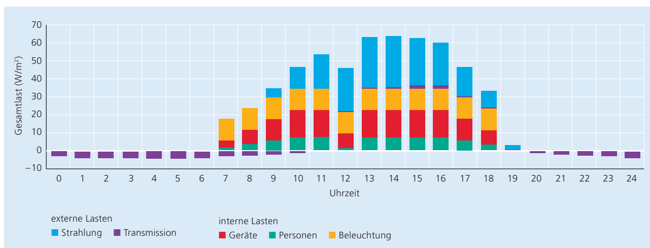
Dynamischer Lastverlauf (24 Stunden, Beispiel 22. September)
