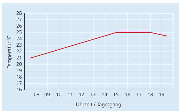
Leitgröße Sollwerttemperatur
