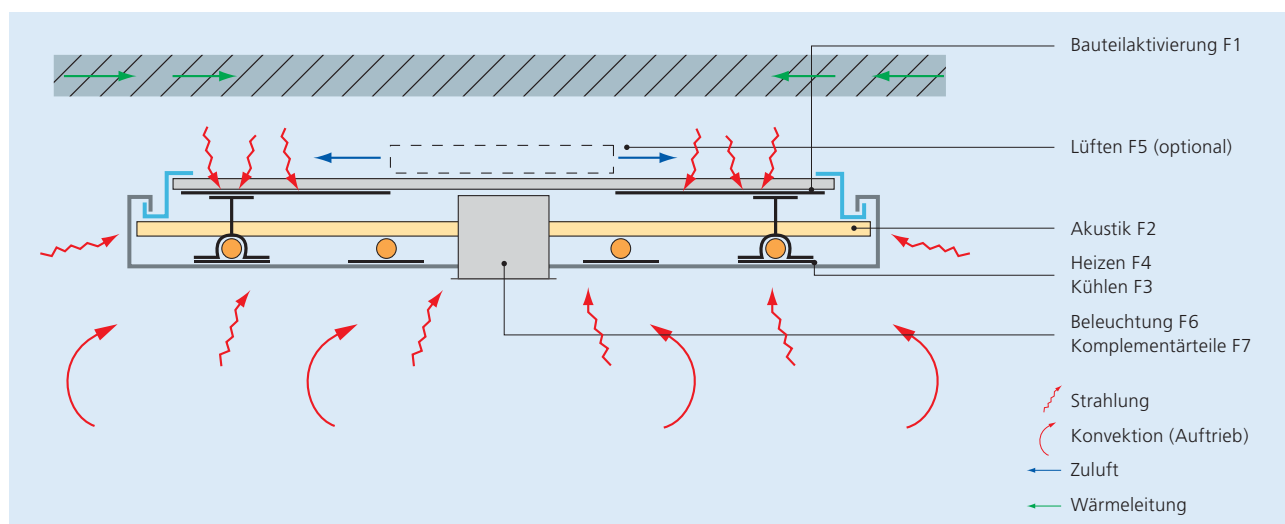
Prinzipanschnitt
