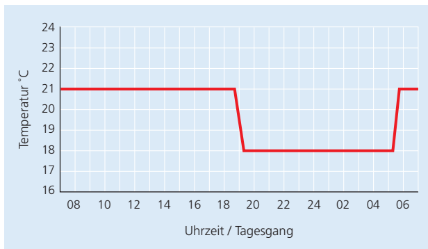
Leitgrösse Sollwerttemperatur
