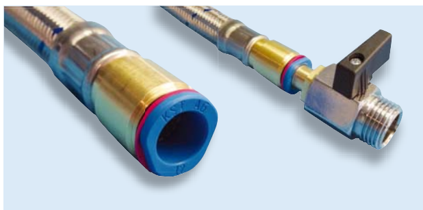
Systemkomponenten mit KST-Spezialsteckkupplung
