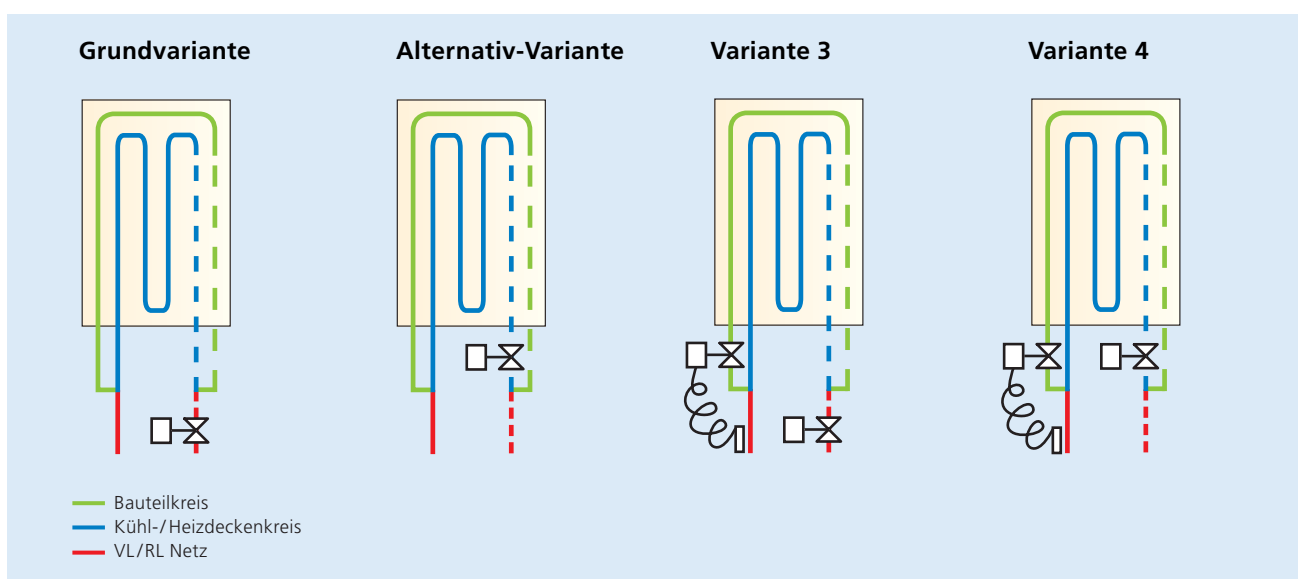
Hydraulische Schaltungen
