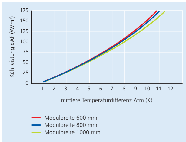
Kühlleistung TBM-System in Abhängigkeit der Modulbreite
